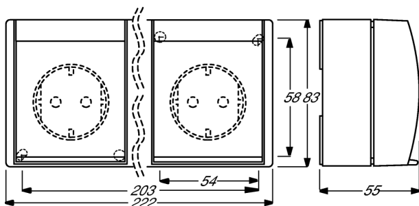
ocean® 3-fach waagrecht SCHUKO® Steckdosen mit Bohrmaßen
