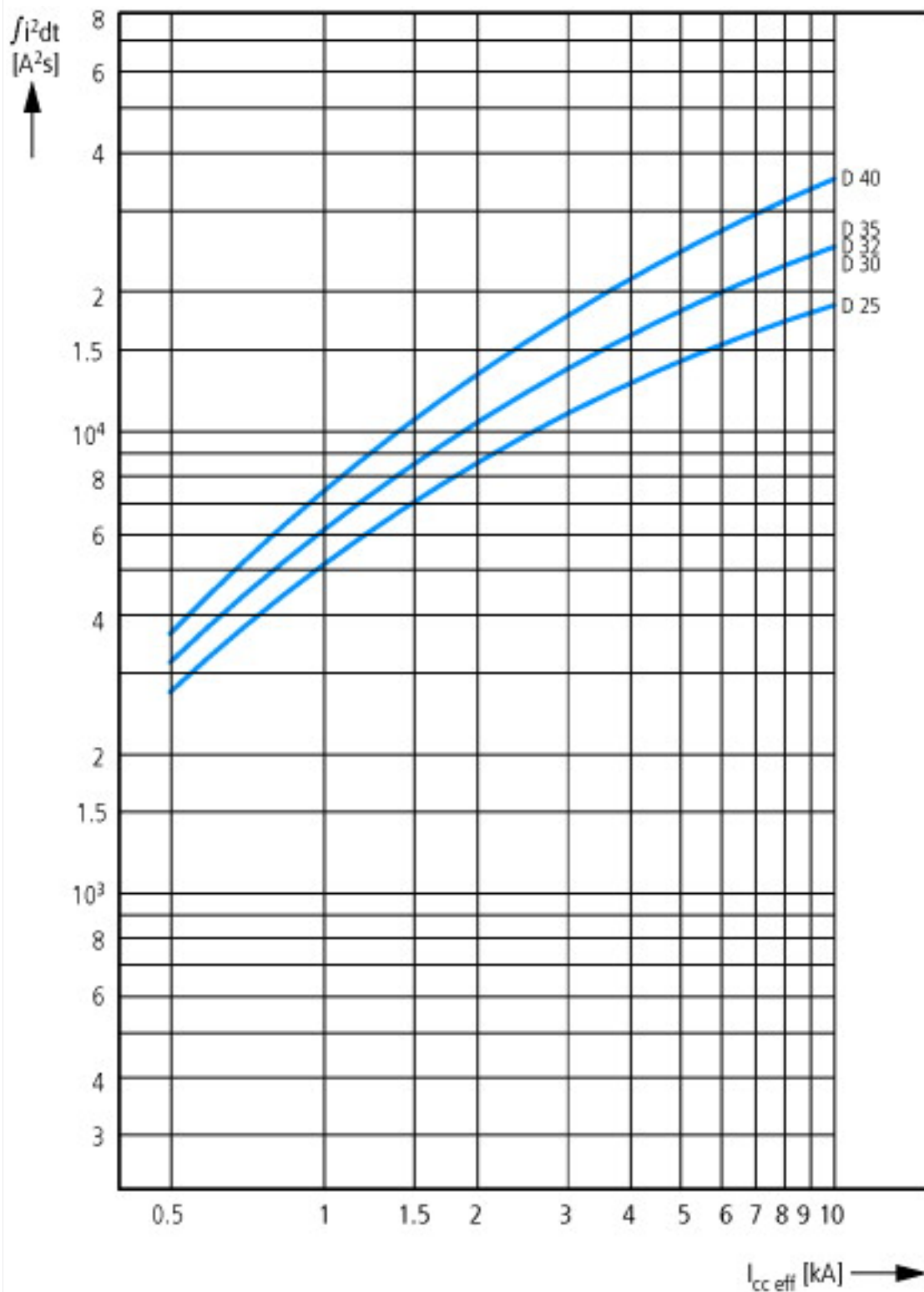
Charakteristik D (25 - 40 A), 240 V
