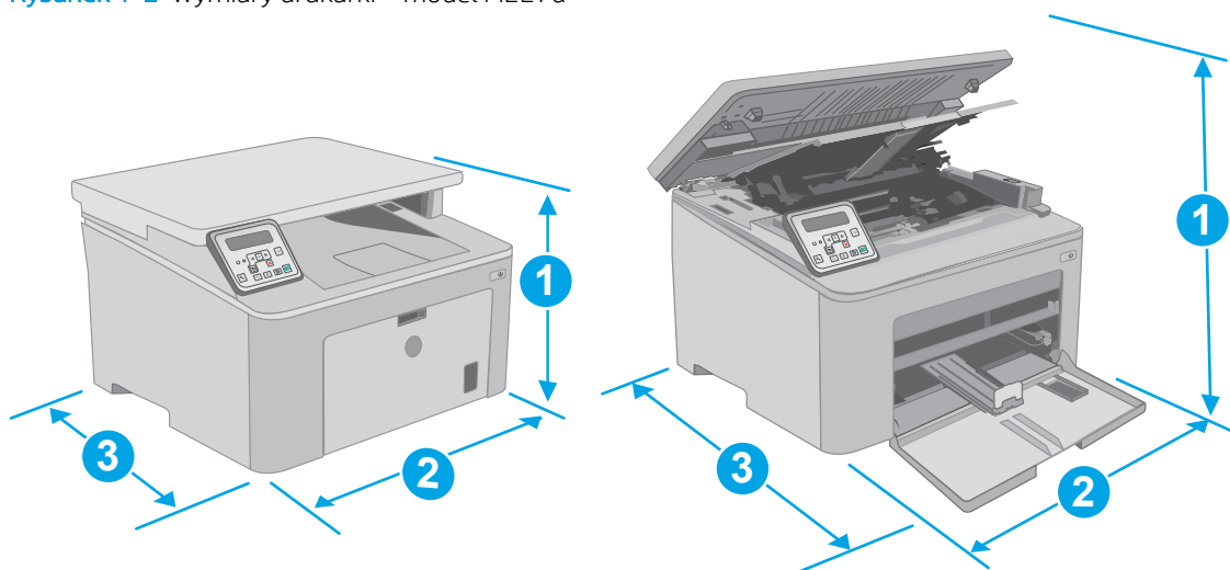
Rysunek 1-2 Wymiary drukarki – model M227d
