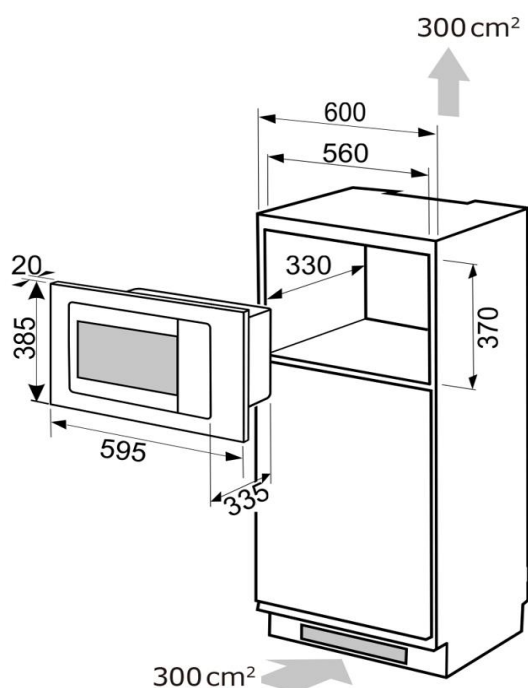
Einbauskizze
