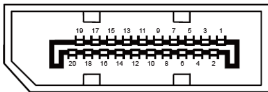
20-poliges Farbdisplay-Signalkabel
