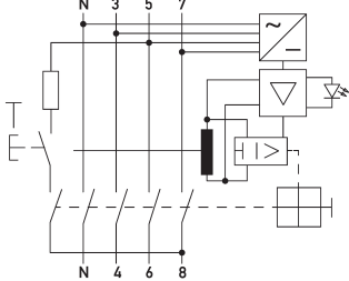
Anschlussschema
