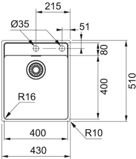
Maris, MRX 210-40 A, Edelstahl, Slimtop / Flächenbündig, Drehknopfventil Edelstahl
