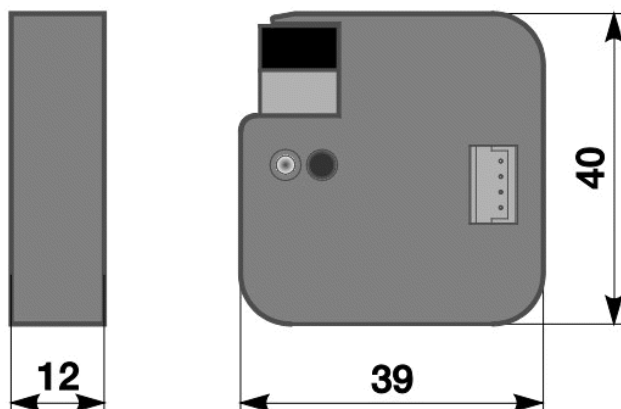
Maßbild
