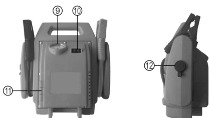
Figure 2 : Vue arrière
