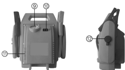
Figura 2: Vista posteriore
