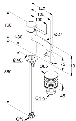
Maßzeichnung
