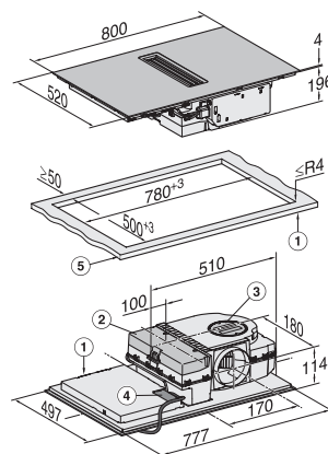
KMDA7272FL, KMDA7473FL – aufliegend – Skizze
