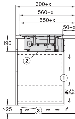
KMDA7272FL, KMDA7473FL – Skizze Seitenansicht aufliegend+X, Plug&Play
