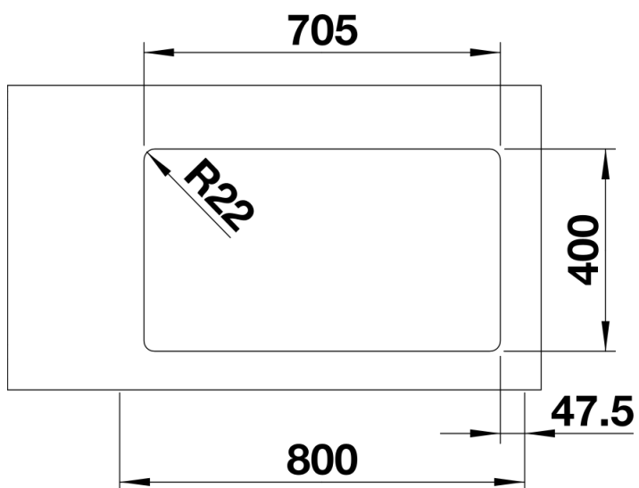
Ausschnitt
