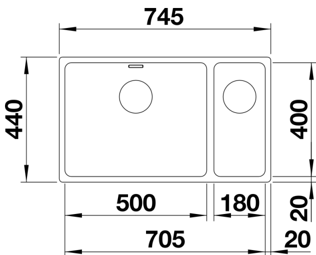
Aufsicht
