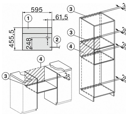
DGC7x40, Skizze
