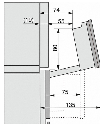
DGC7x4x, DGC7x4x-55, DGC7xxx, Skizze
