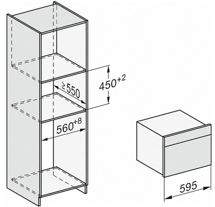
DGC7x4x, DGC7x4xX Skizze
