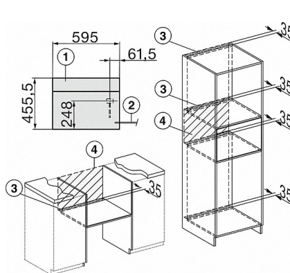
DGC7x40, Skizze
