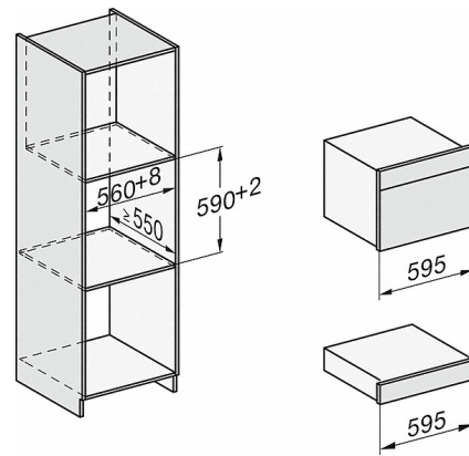
ESW7x10, Skizze
