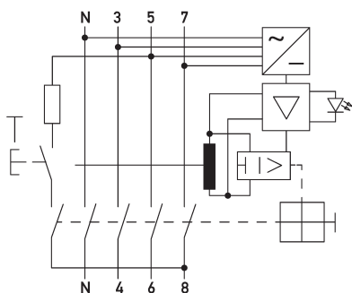
Schaltungsbeispiel Fehlerstromschutzschalter DFS 4 040-4/0,30-B NK S
