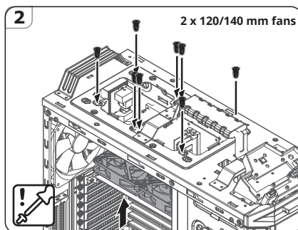
2.7.4 Install bottom fan (2 x 120mm fans)
