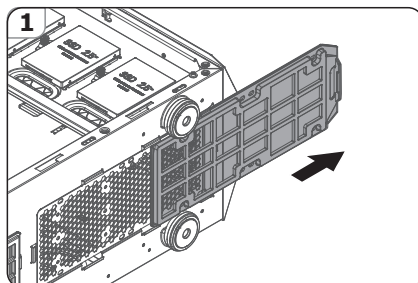
2.7.4 Install bottom fan (2 x 120mm fans)
