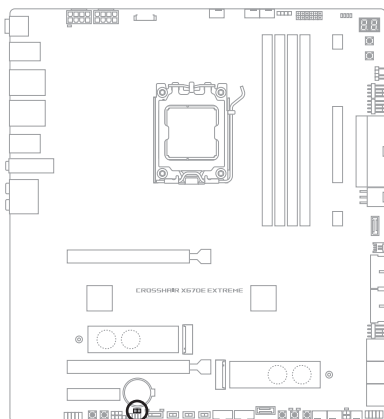
T_SENSOR
