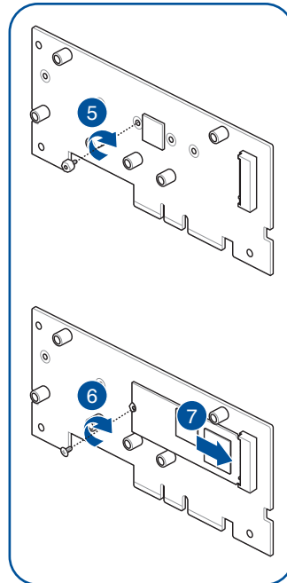
Rückseite
