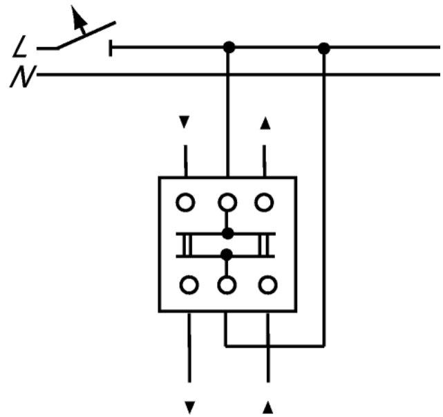
Jalousieschalter-taster, 1 P+N+PE, Drehgriff oder Schlüssel 2713-... und 2733-...
