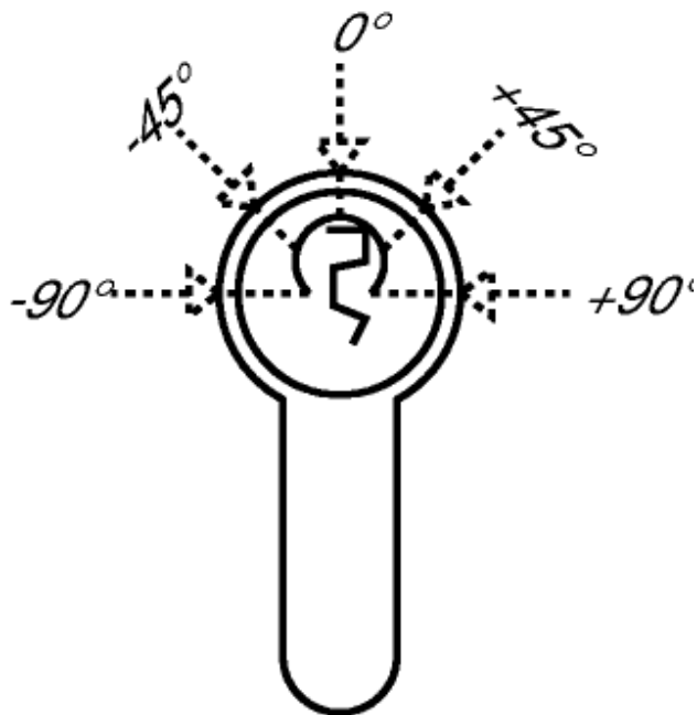
mögliche Bartstellung des DIN-Halbzylingerschlosses bei Jalousieschaltern
