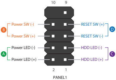
Systemblende-Stiftleiste
