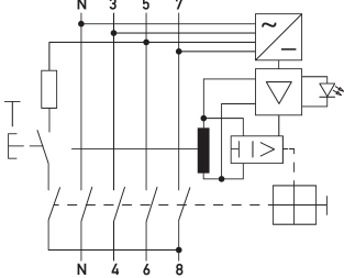
Anschlusschema
