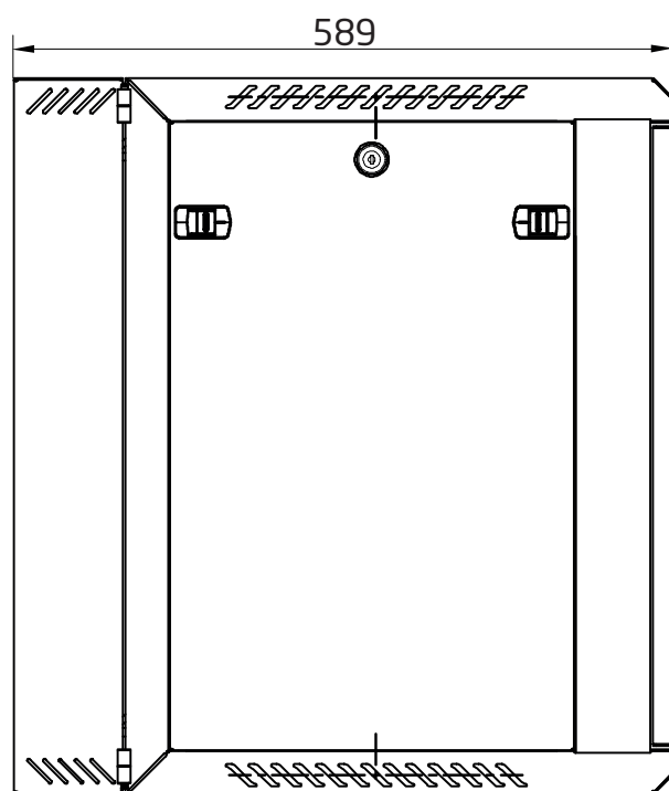
Seiteninnenansicht
