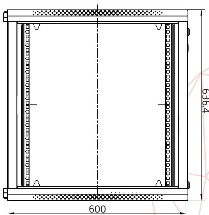
Vorderseiteninnenansicht
