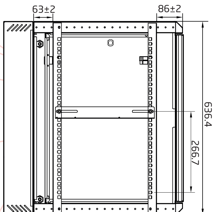
Seiteninnenansicht
