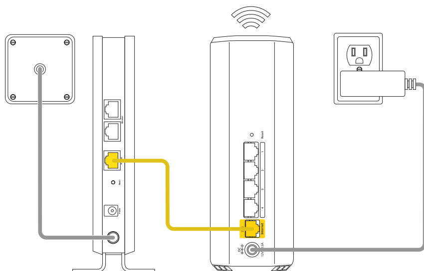
Abbildung 5: Verkabeln des Routers
