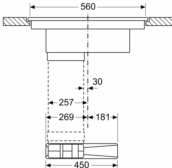
Maße in mm Frontansicht
