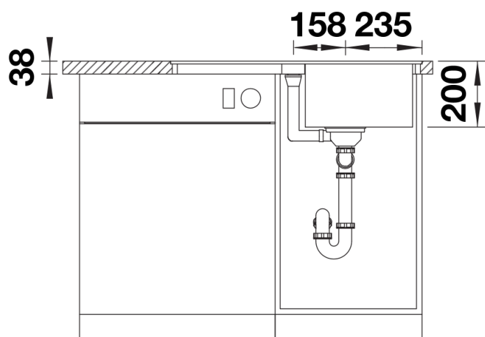
Frontansicht
