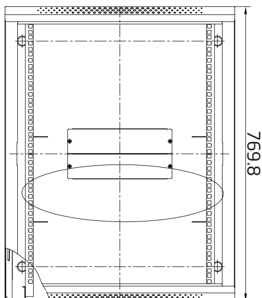
Seiteninnenansicht
