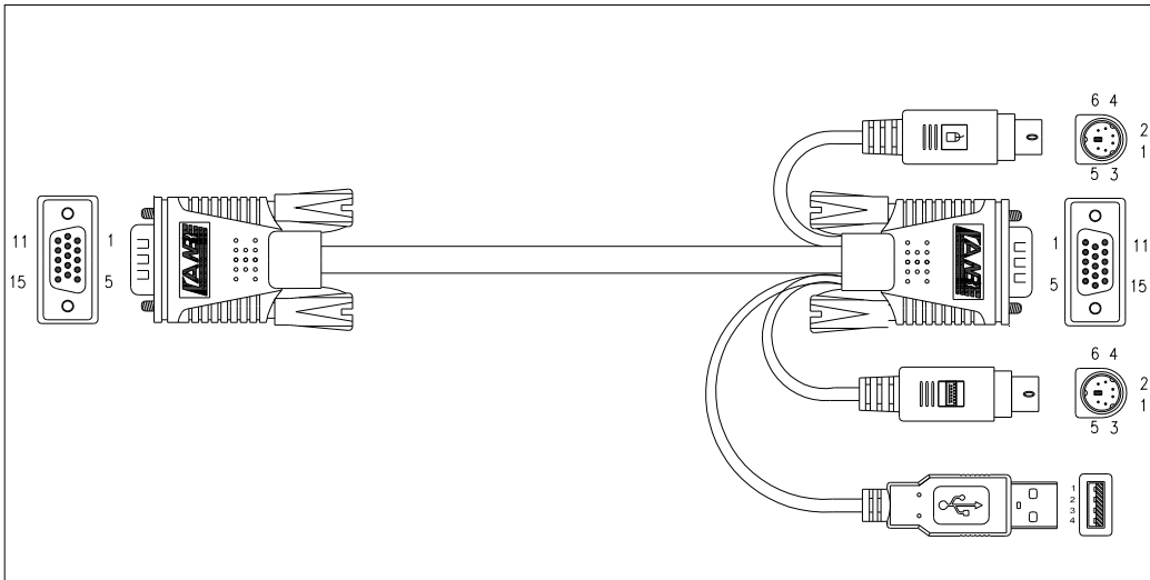
USB- und PS/2-Verbindungskabel
