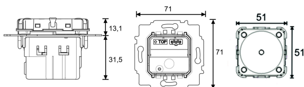
Maßbild
