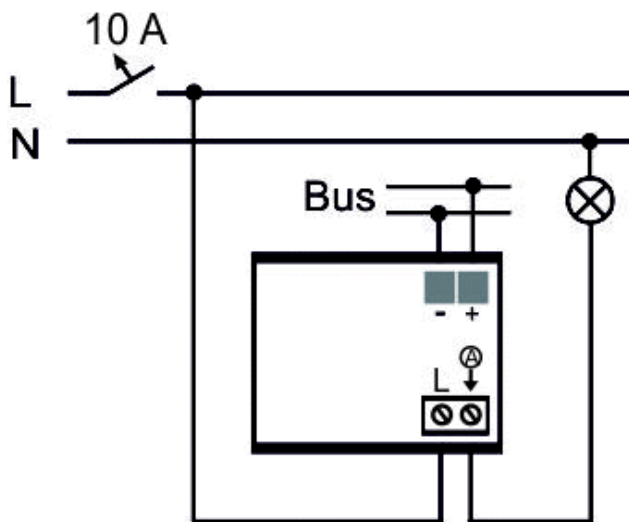
Anschlussbild
