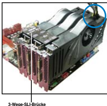
3-Wege-SLI-Brücke
