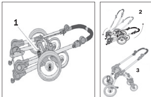
Zamknutie výkyvu
