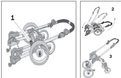
Šarnyro fiksavimas
