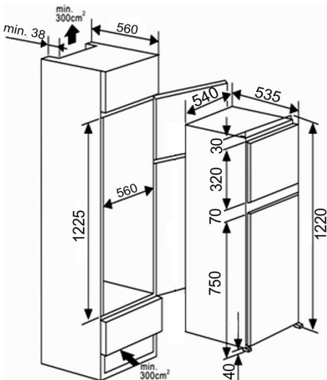
Einbauskeizze
