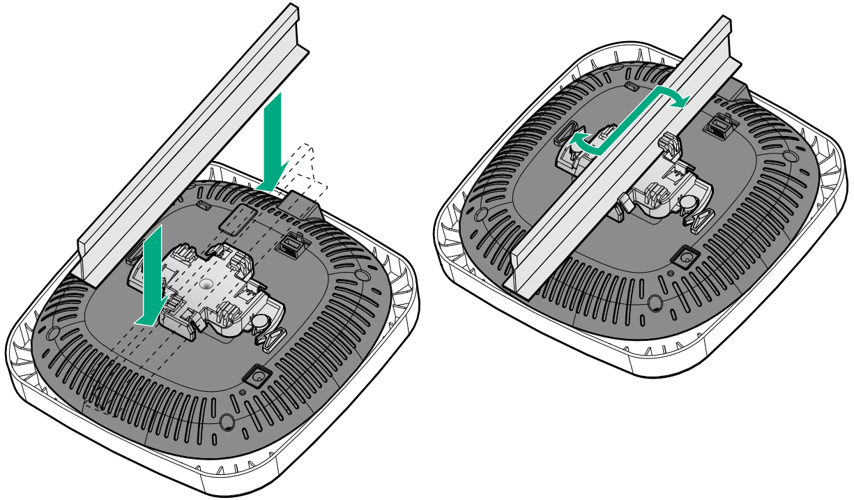
Abbildung 6 Montieren des AP an einer 9/16-Zoll-Deckenschiene
