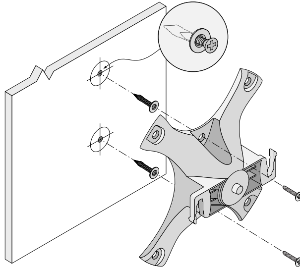
Abbildung 8 Befestigen der Halterung an einer Wand (alternative Anbringung)
