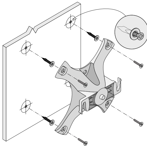
Abbildung 7 Befestigen der Halterung an einer Wand
