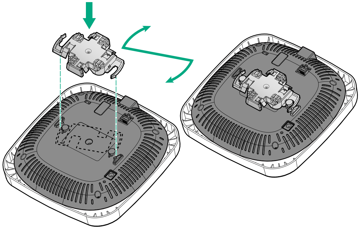
Abbildung 4 Anbringen der Deckenmontagehalterung am AP
