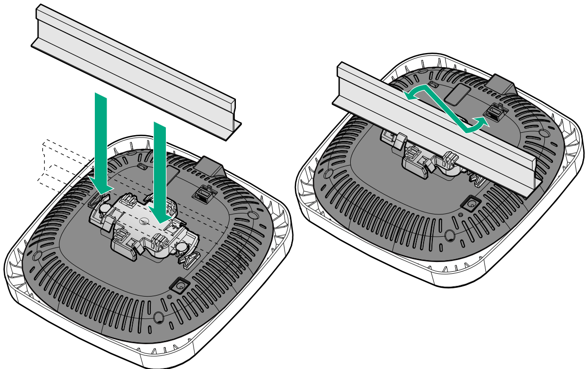
Abbildung 5 Montieren des AP an einer 15/16-Zoll-Deckenschiene
