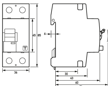
Maßzeichnung Fehlerstromschutzschalter DFS 2 025-2/0,30-HP
