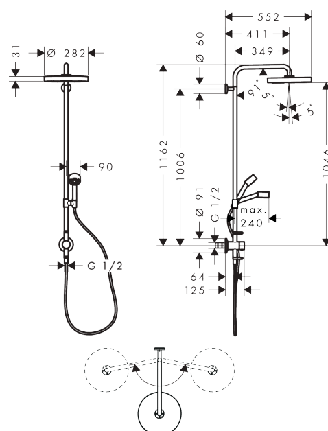
Maßzeichnung
