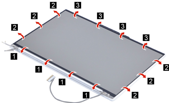
Figure 27. Remove the LCD bezel
