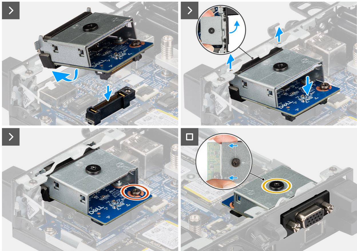
Abbildung 50. Einbauen des VGA-Moduls
