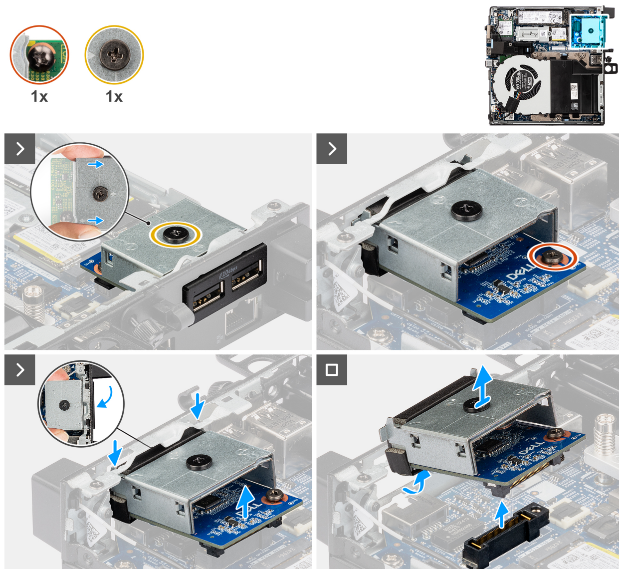
Abbildung 38. Entfernen des dualen USB-3.2-Gen2-Moduls
