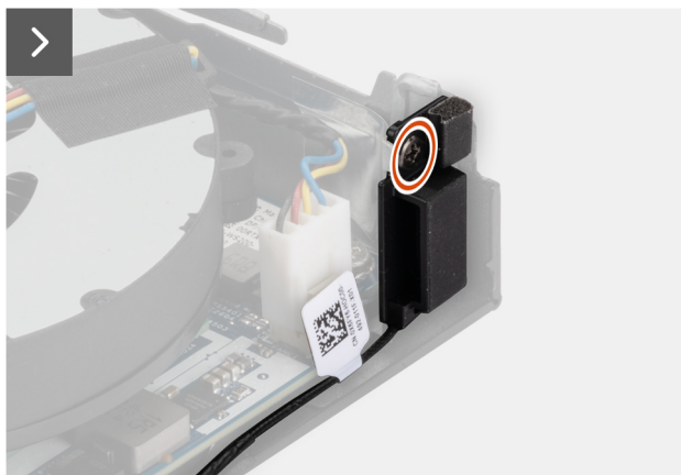
Abbildung 66. Entfernen des Antennenmoduls (schwarzes Kabel)
