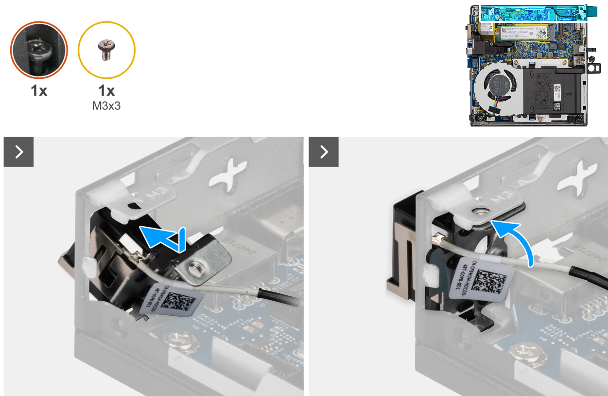
Abbildung 64. Einbauen des Antennenmoduls (weißes Kabel)
