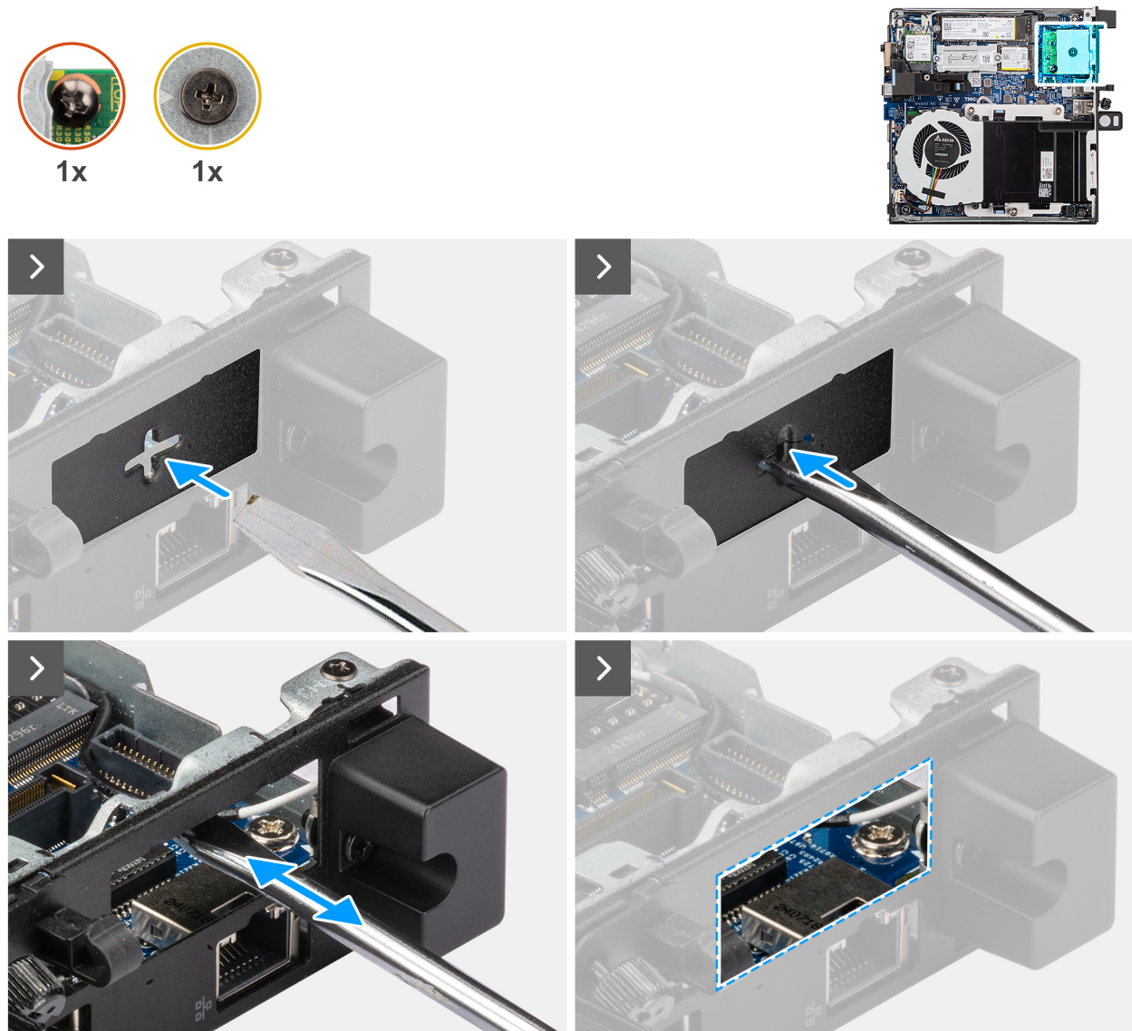
Abbildung 39. Installieren des dualen USB-3.2-Gen2-Moduls
