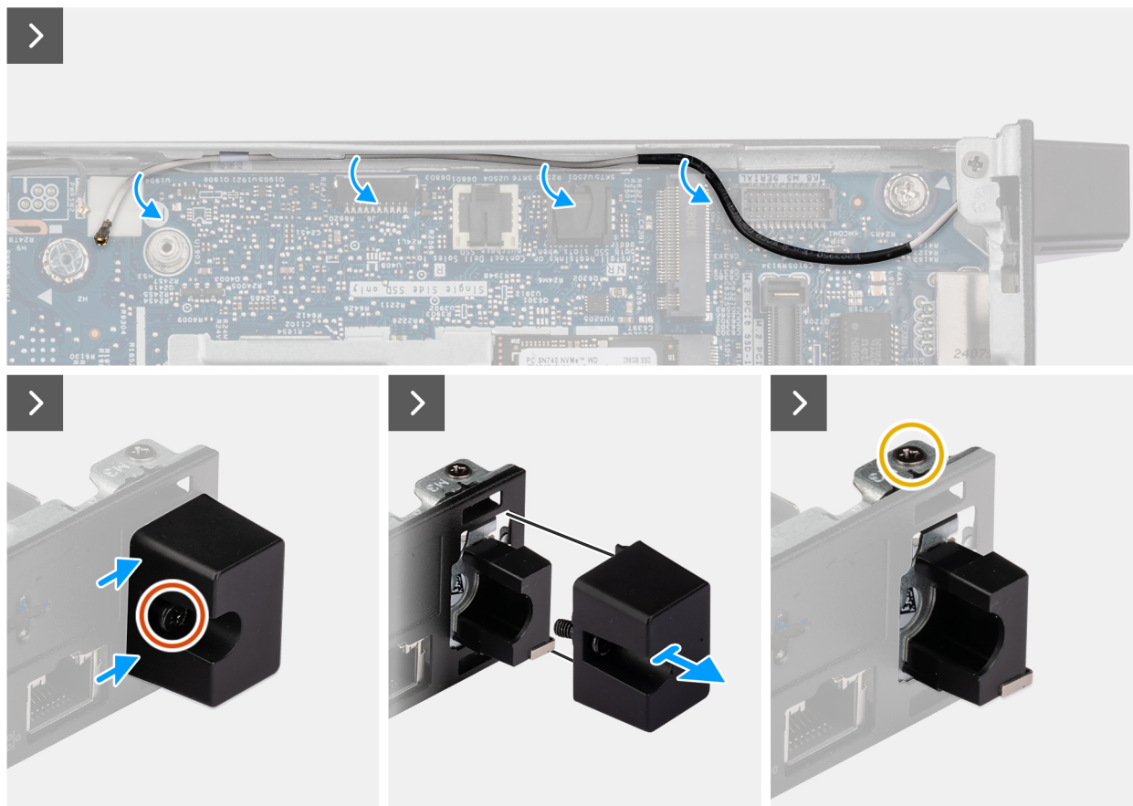
Abbildung 62. Entfernen des Antennenmoduls (weißes Kabel)
