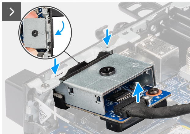
Abbildung 51. Entfernen des PS2-Moduls
