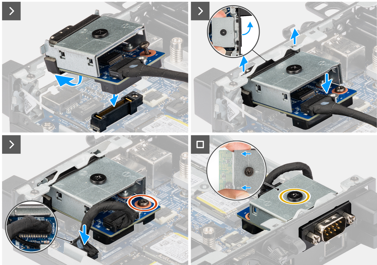
Abbildung 56. Installieren des seriellen Moduls
