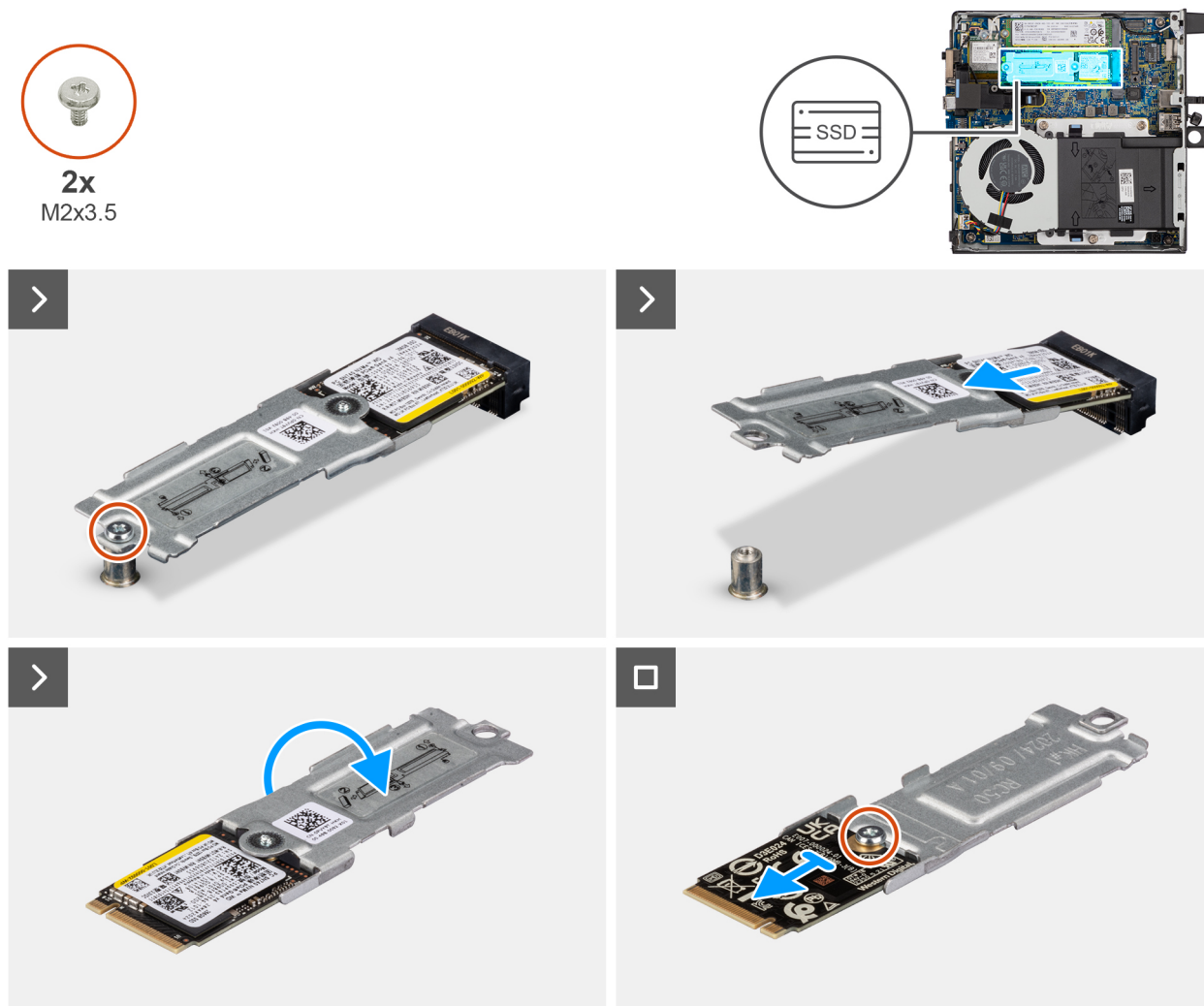
Abbildung 16. Entfernen des 2230-Solid-State-Laufwerks
