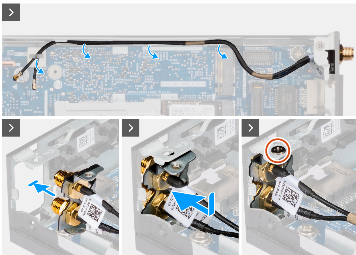
Abbildung 37. Installieren des SMA-Antennenmoduls
