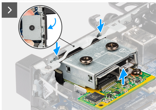
Abbildung 57. Entfernen des Glasfasermoduls
