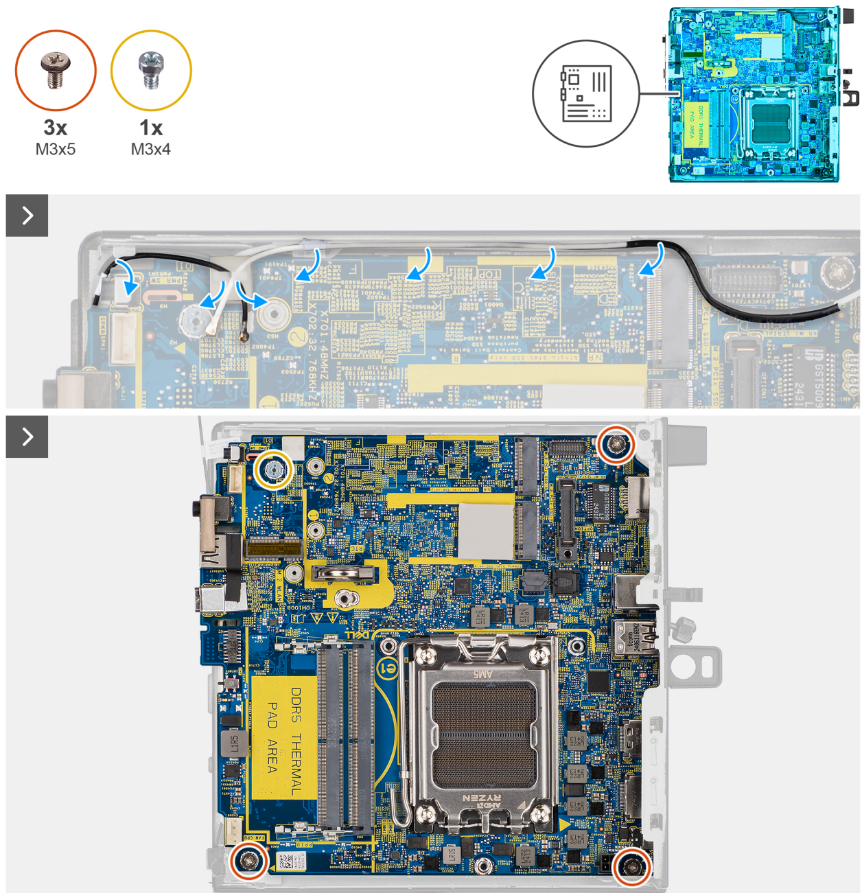
Abbildung 73. Entfernen der Systemplatte
