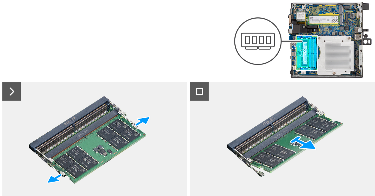
Abbildung 32. Entfernen des Arbeitsspeichermoduls
