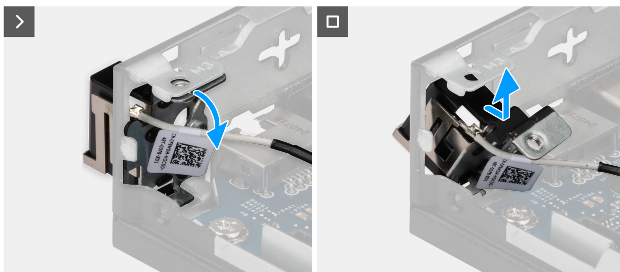
Abbildung 63. Entfernen des Antennenmoduls (weißes Kabel)
