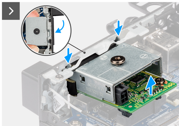
Abbildung 41. Entfernen des USB-Type-C-Moduls
