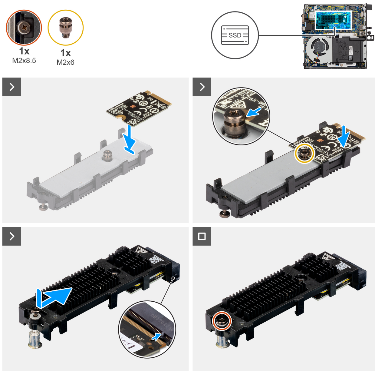
Abbildung 23. Einbauen des M.2 2230-PCIe-SSD-Laufwerks
