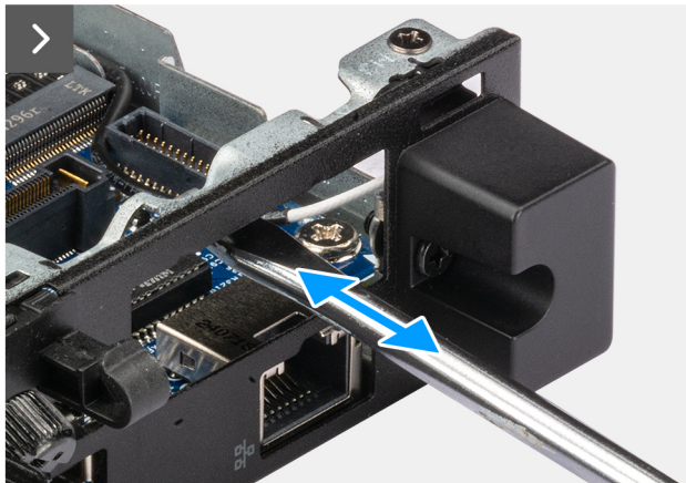
Abbildung 52. Installieren des PS2-Moduls
