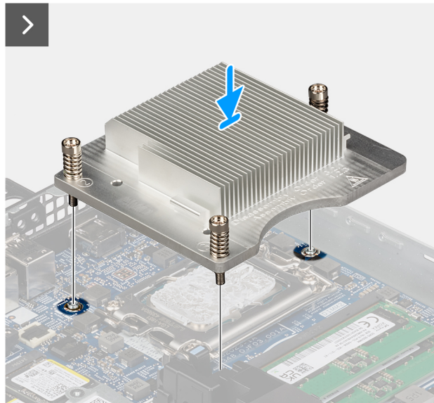
Abbildung 61. Einsetzen des Kühlkörpers
