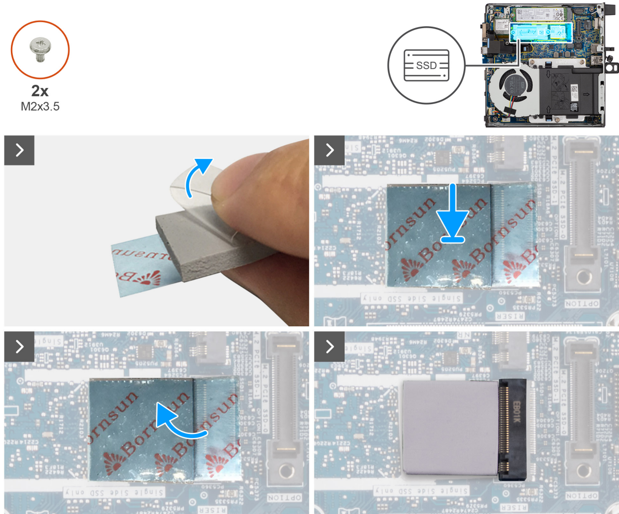
Abbildung 17. Einbauen des 2230-Solid-State-Laufwerks
