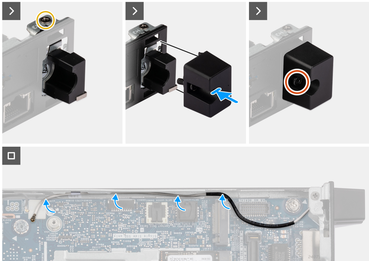
Abbildung 65. Einbauen des Antennenmoduls (weißes Kabel)
