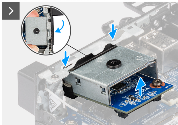
Abbildung 45. Entfernen des HDMI-Moduls
