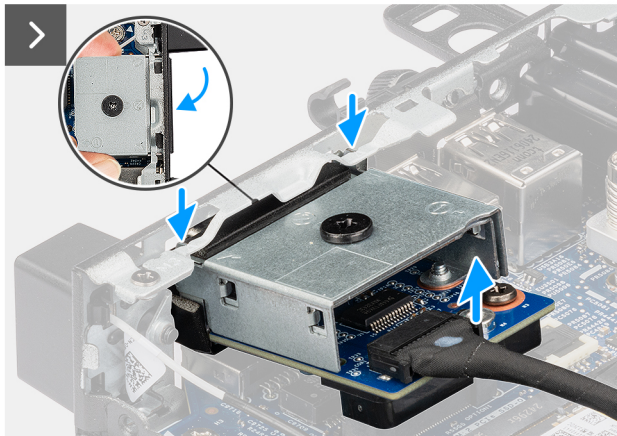
Abbildung 54. Entfernen des seriellen Moduls
