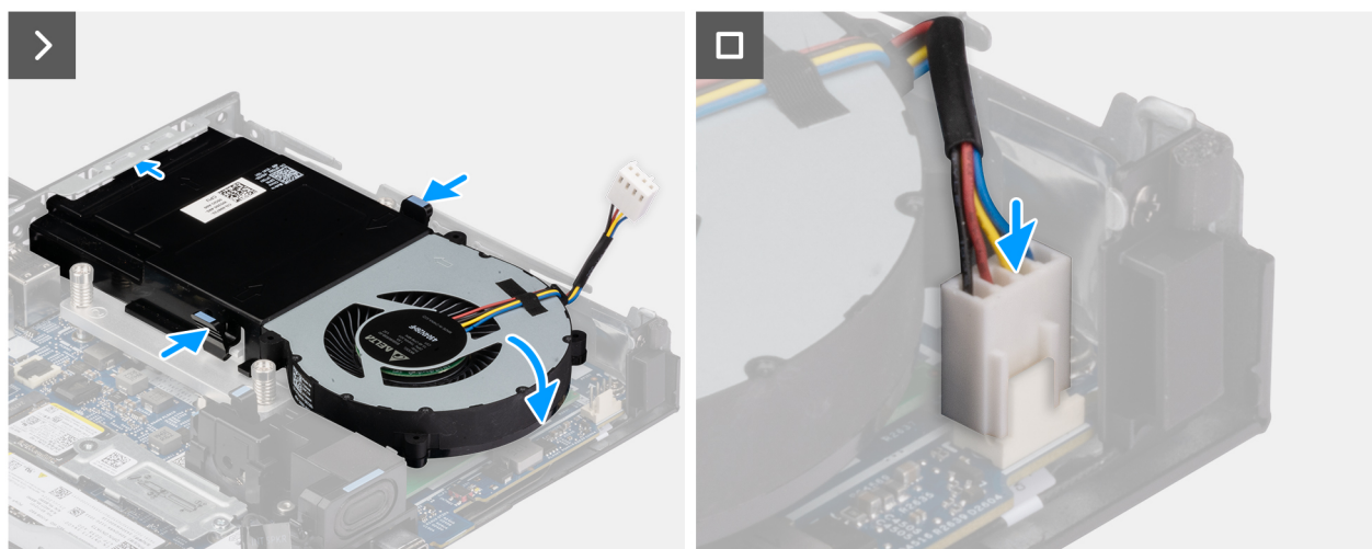
Abbildung 31. Einbauen des Lüfters
