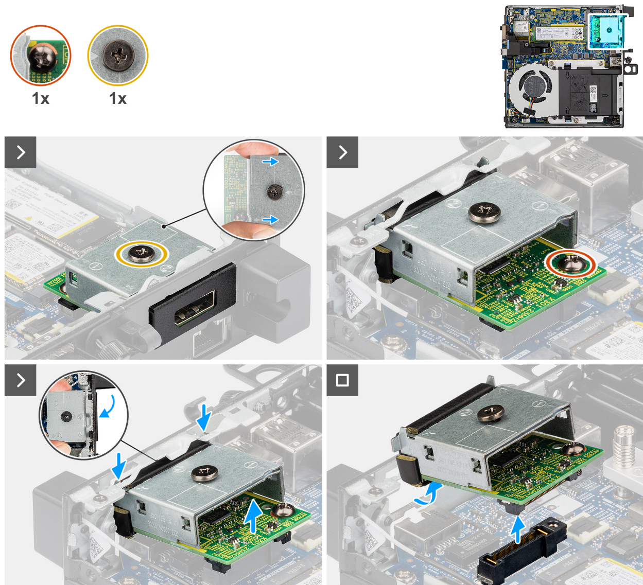
Abbildung 42. Entfernen des DisplayPort-Moduls
