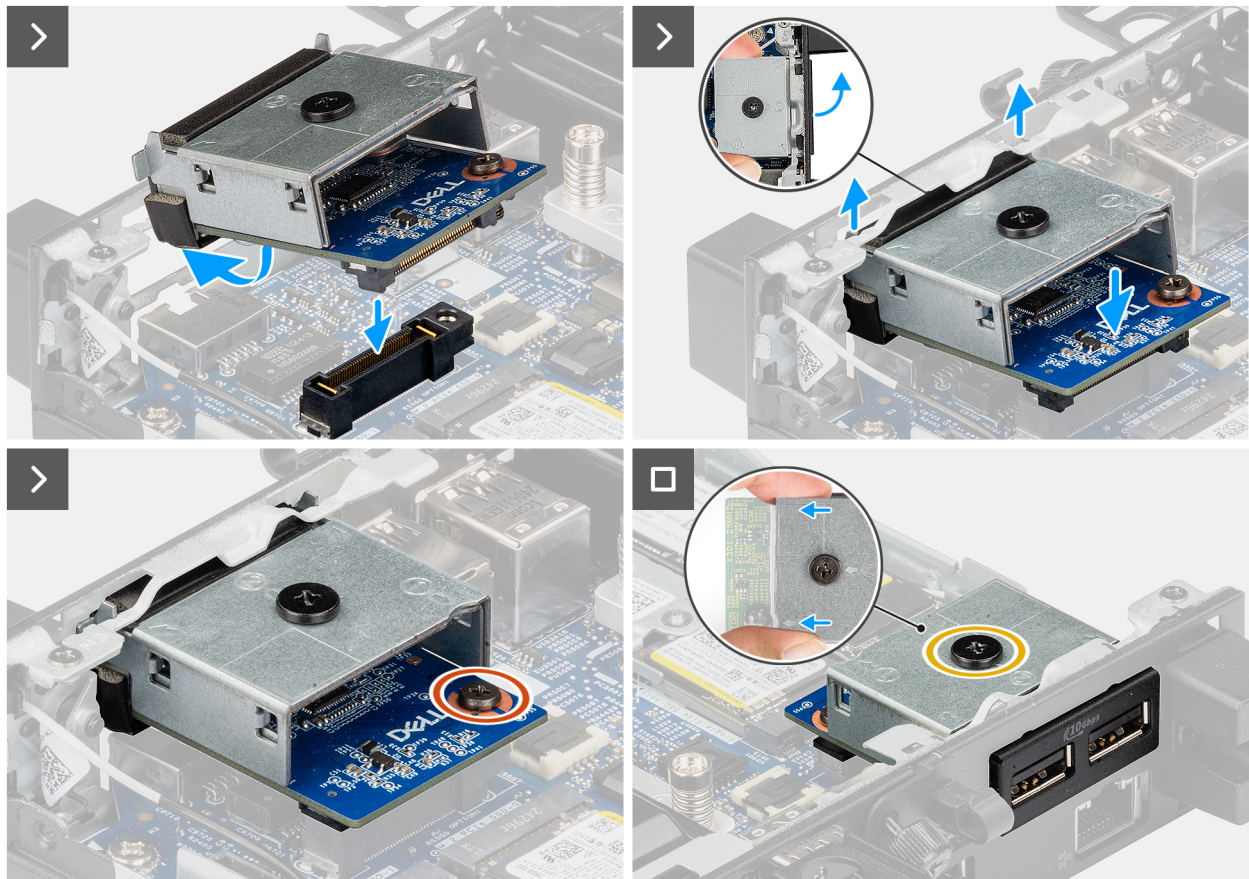
Abbildung 40. Installieren des dualen USB-3.2-Gen2-Moduls
