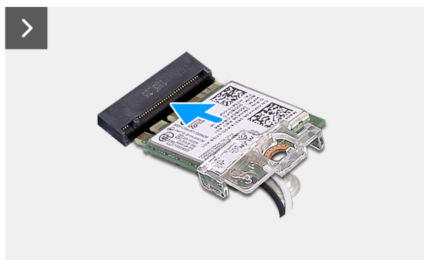
Abbildung 27. Installieren der Wireless-Karte
