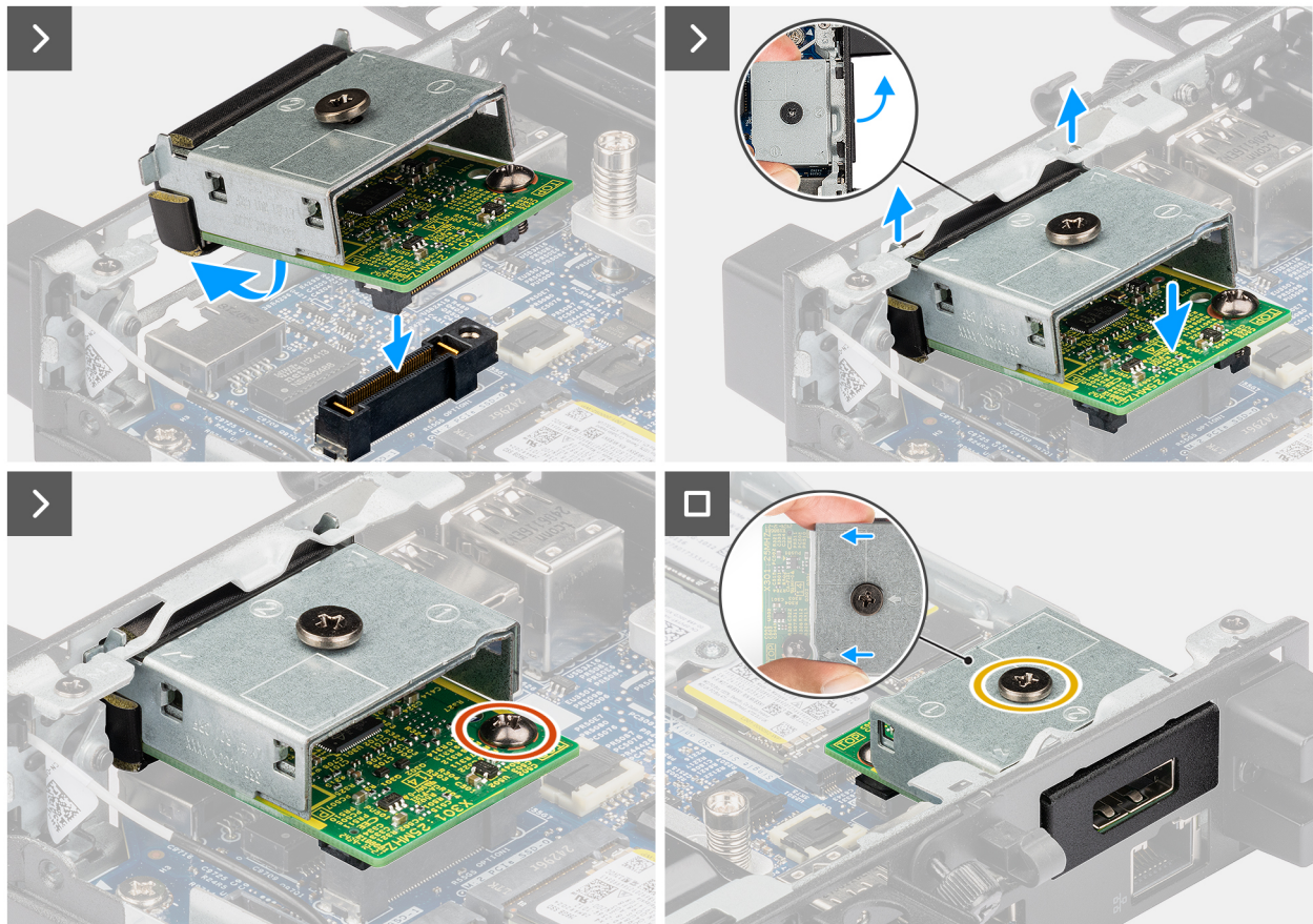
Abbildung 44. Einbauen des DisplayPort-Moduls
