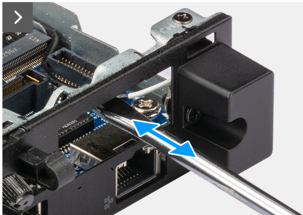
Abbildung 49. Einbauen des VGA-Moduls
