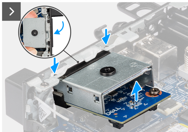
Abbildung 48. Entfernen des VGA-Moduls
