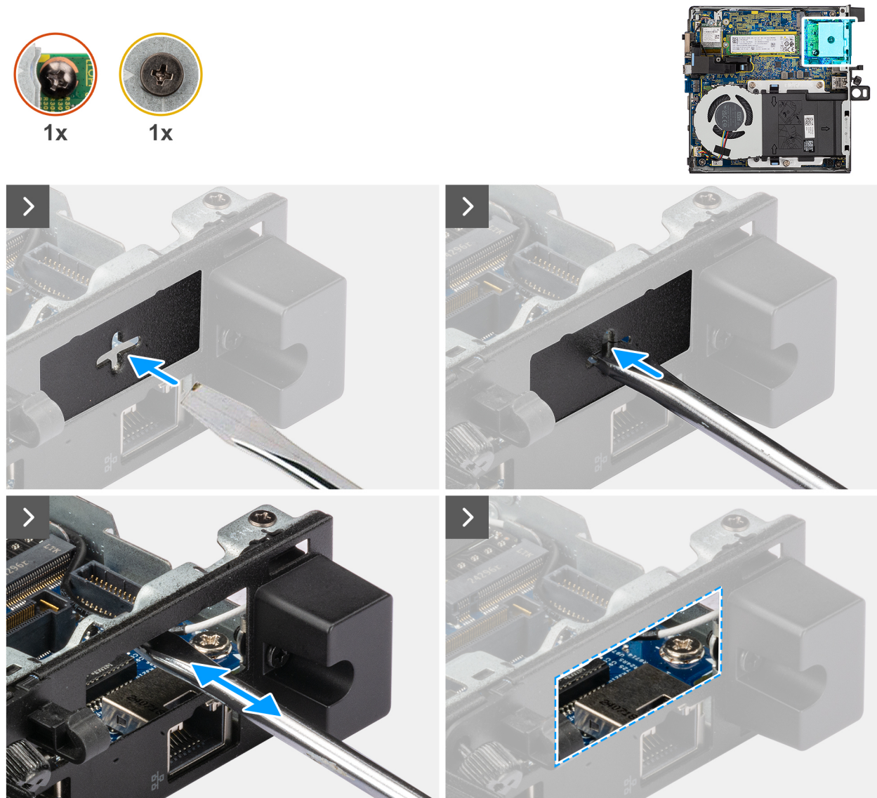
Abbildung 43. Einbauen des DisplayPort-Moduls
