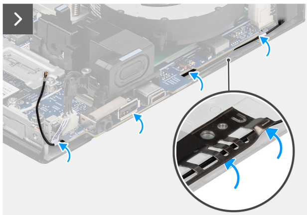
Abbildung 67. Einbauen des Antennenmoduls (schwarzes Kabel)
