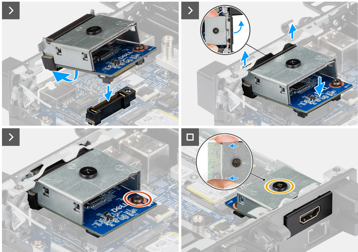
Abbildung 47. Einbauen des HDMI-Moduls
