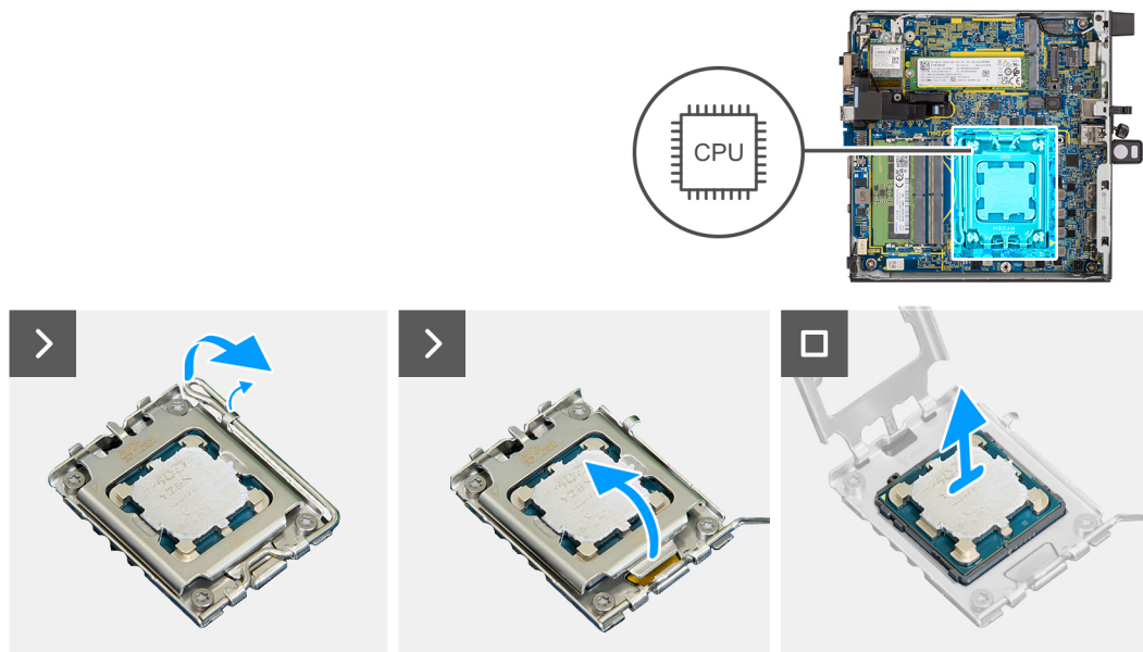
Abbildung 68. Entfernen des Prozessors
