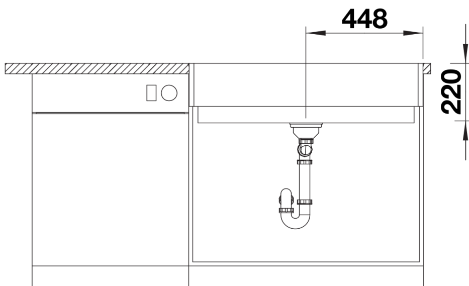
Frontansicht
