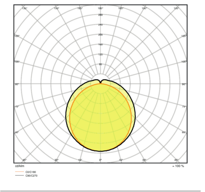
LVK Polar
