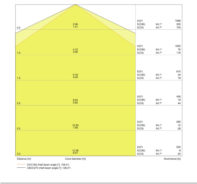
LVK Kegel
