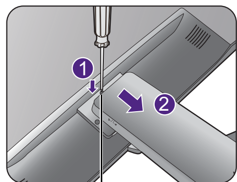
Auslösetaste
