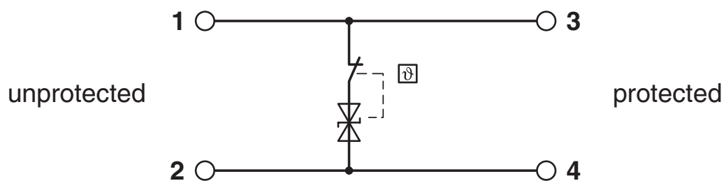
Schaltplan
