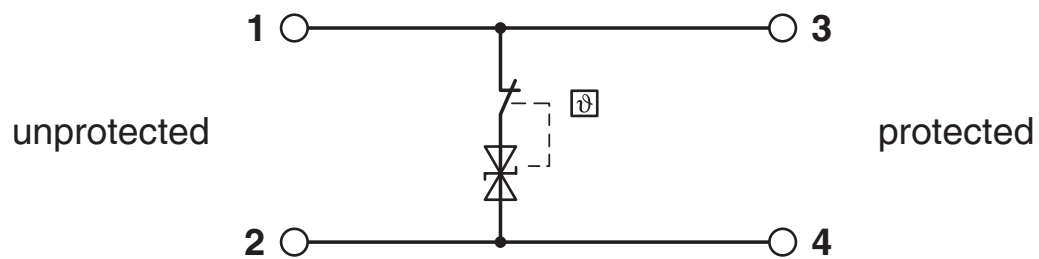
Schaltplan
