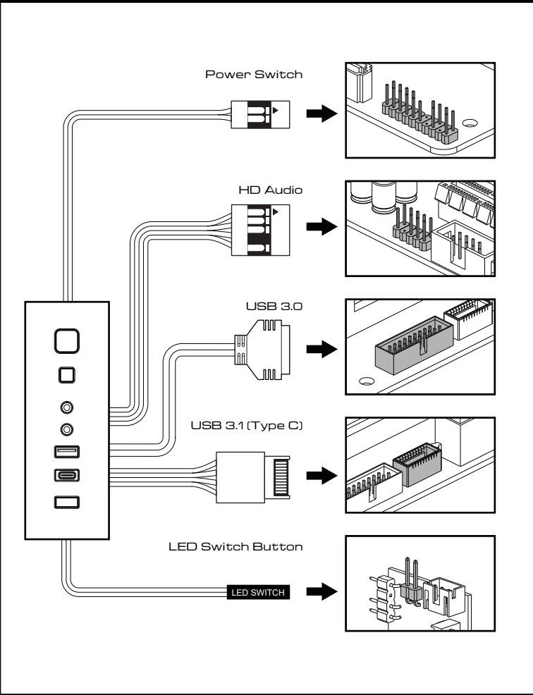
▼ I/O cables
