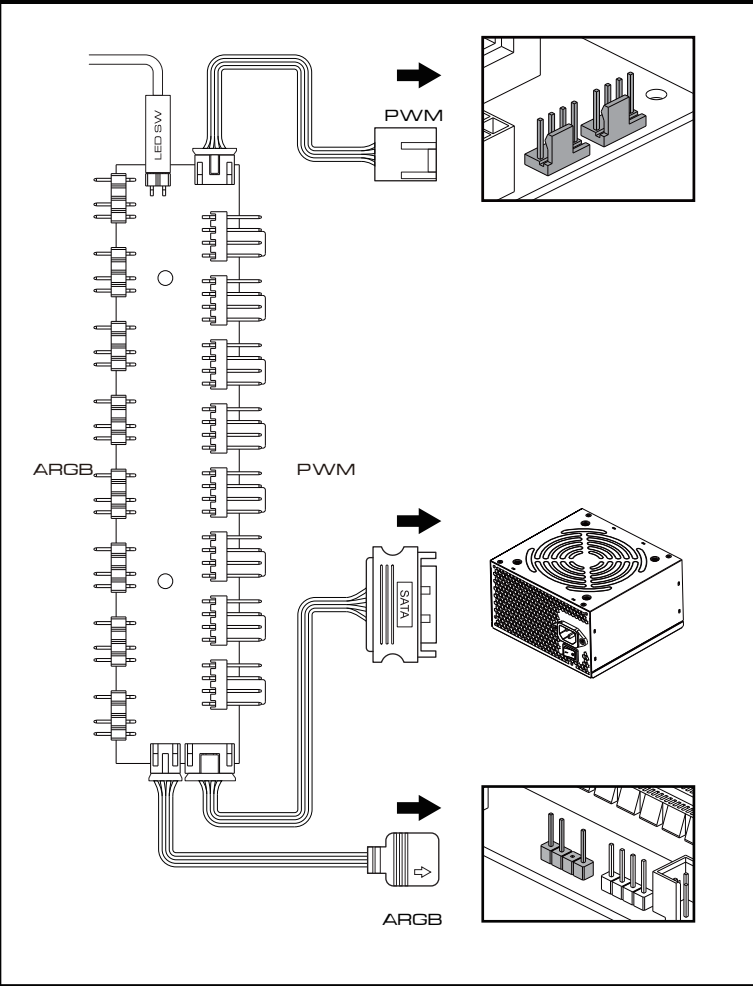
▼ Fan Hub
