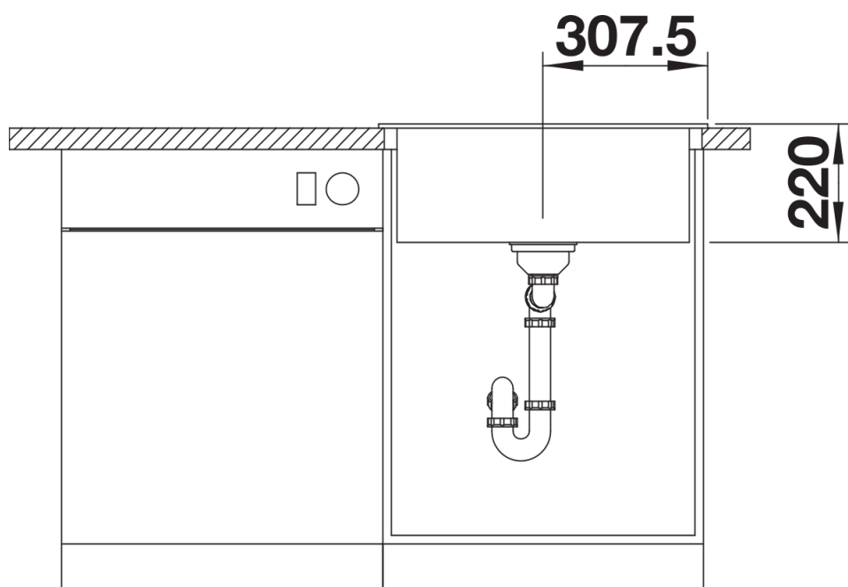
Frontansicht
