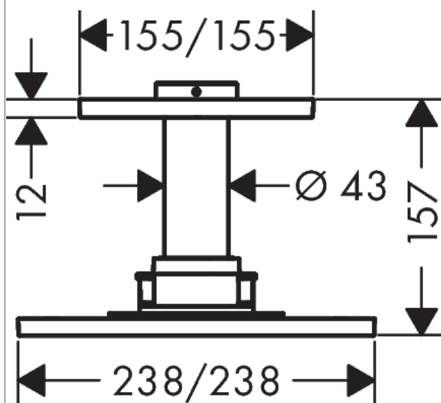
Maßzeichnung
