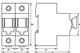
Maßzeichnung Gruppenansicht
