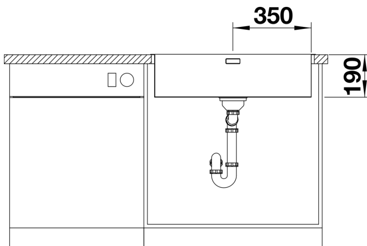
Frontansicht
