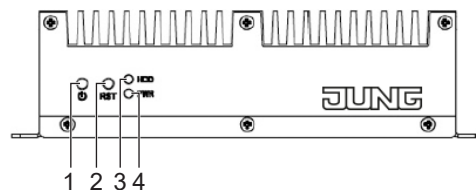
Abb. 1: Gerät Vorderseite
