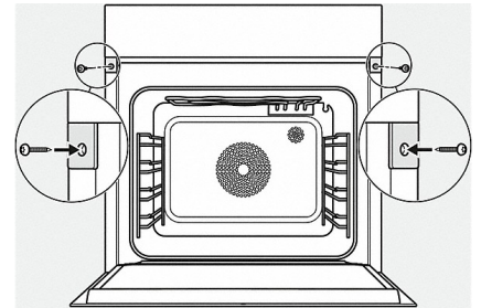
DGC7x6x, DGC7x6xX Skizze
