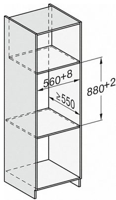
ESW7x20, Skizze
