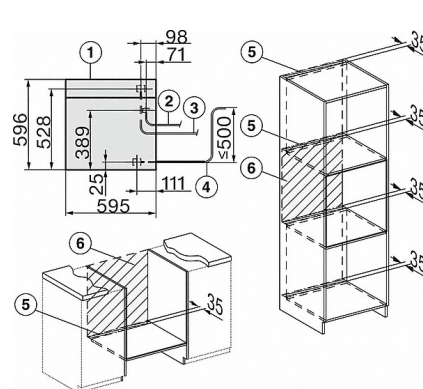
DGC7x65, DGC7x65X Skizze
