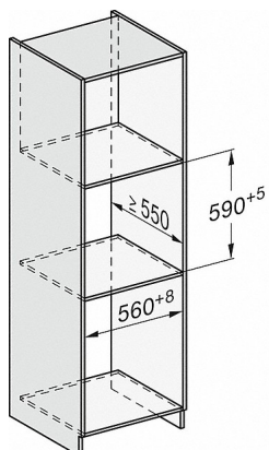
DGC7x6x, DGC7x6xX Skizze
