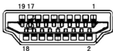
19-poliges Farbdisplay-Signalkabel
