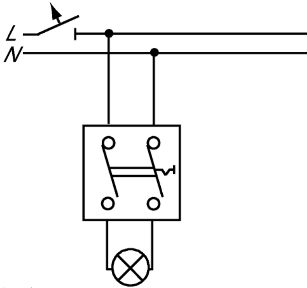
Aus 2-polig
